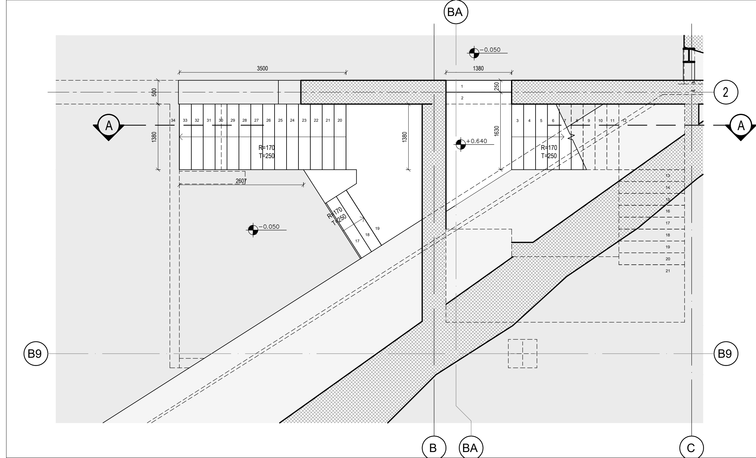
Plani i nivelit f.f. +3.87 Shkalla 1 : 50
