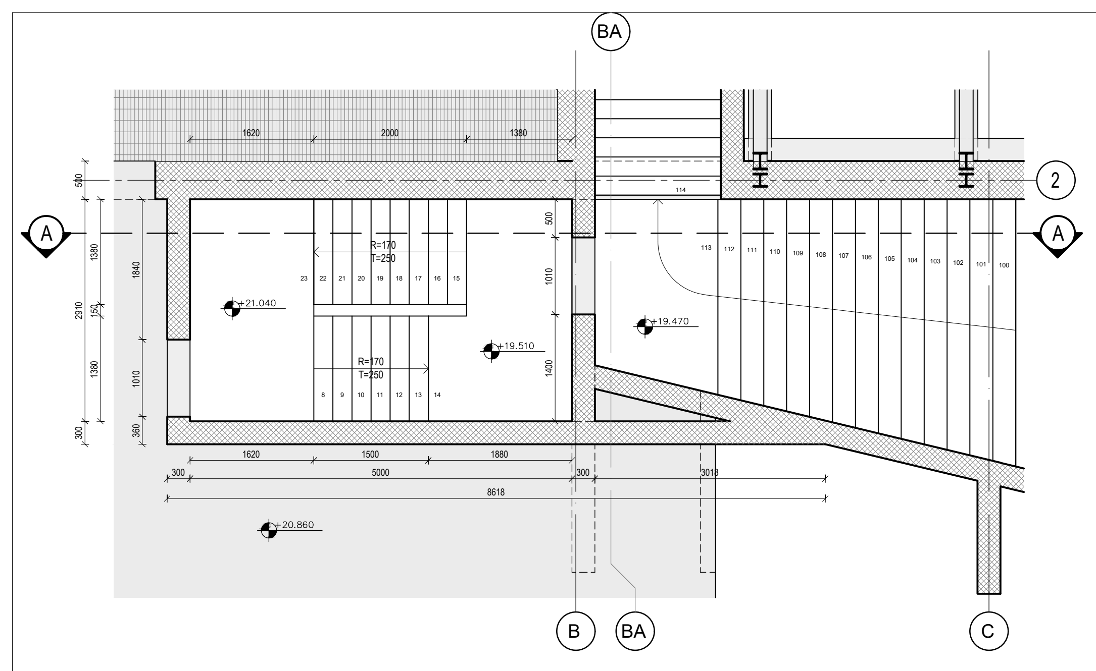
Plani i nivelit f.f. +21.04 Shkalla 1 : 50
