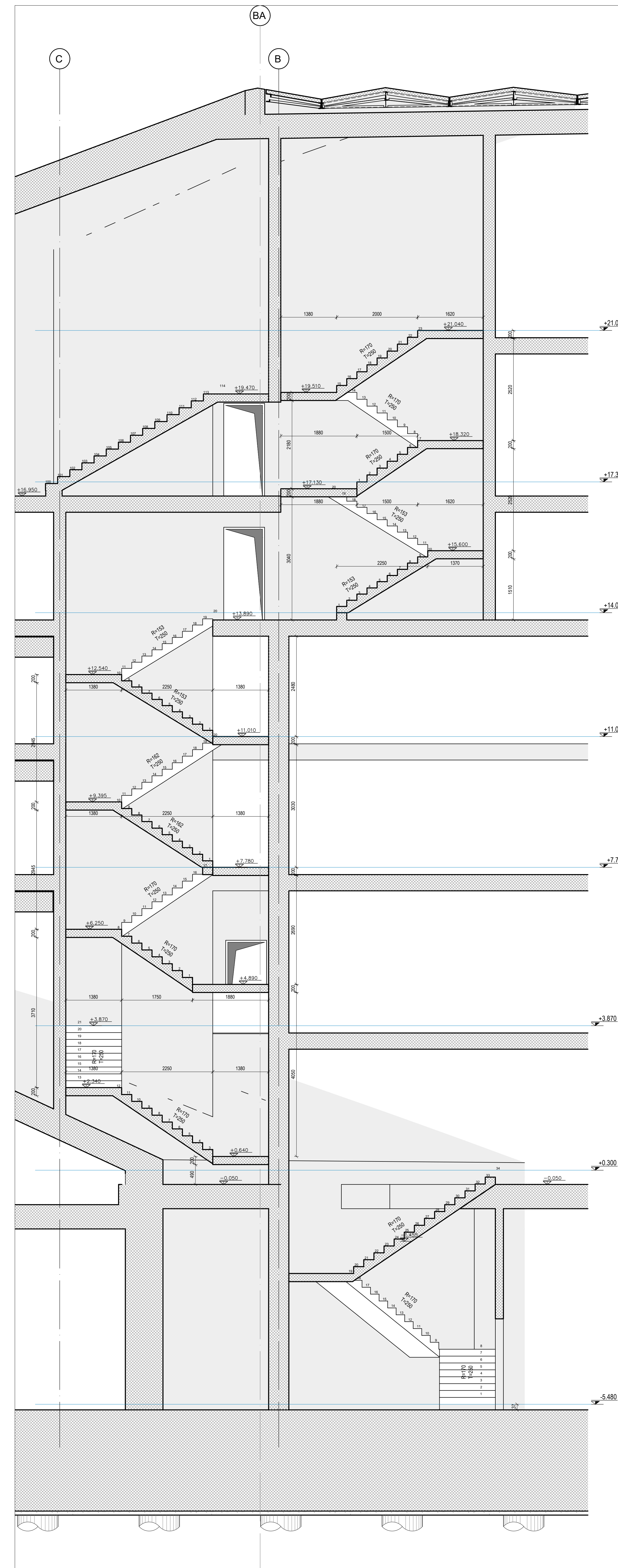
Seksioni A-A Shkalla 1 : 50
