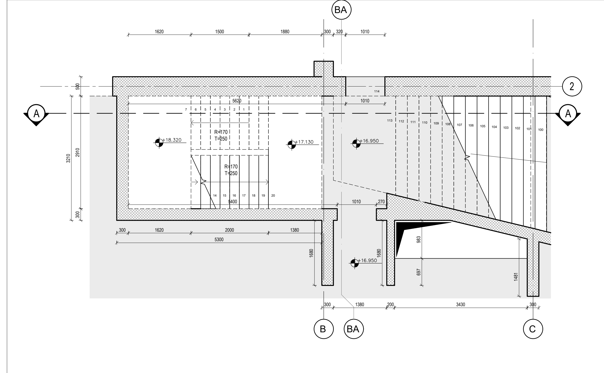
Plani i nivelit f.f. +17.30 Shkalla 1 : 50
