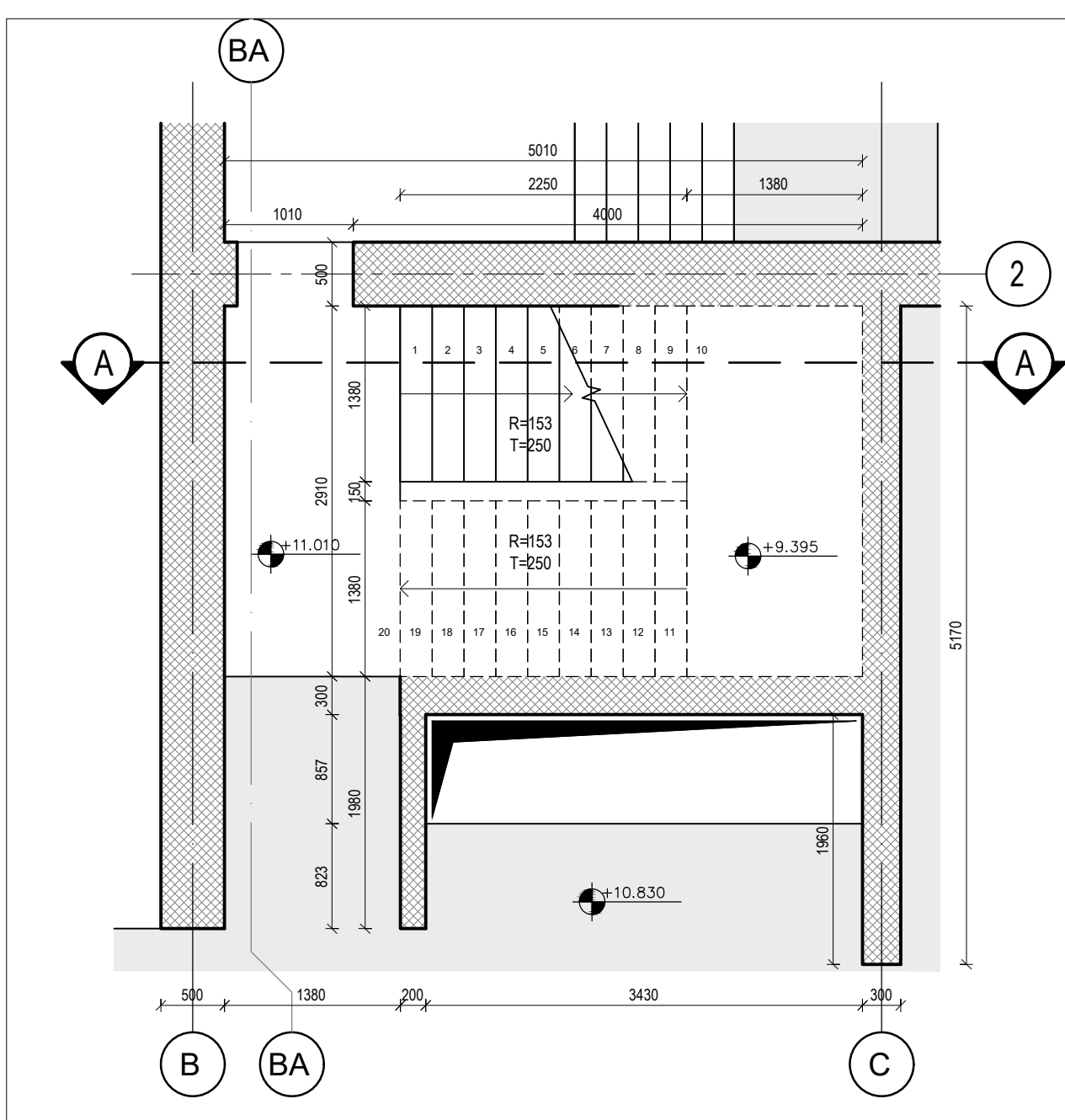
Plani i nivelit f.f. +11.01 Shkalla 1 : 50
