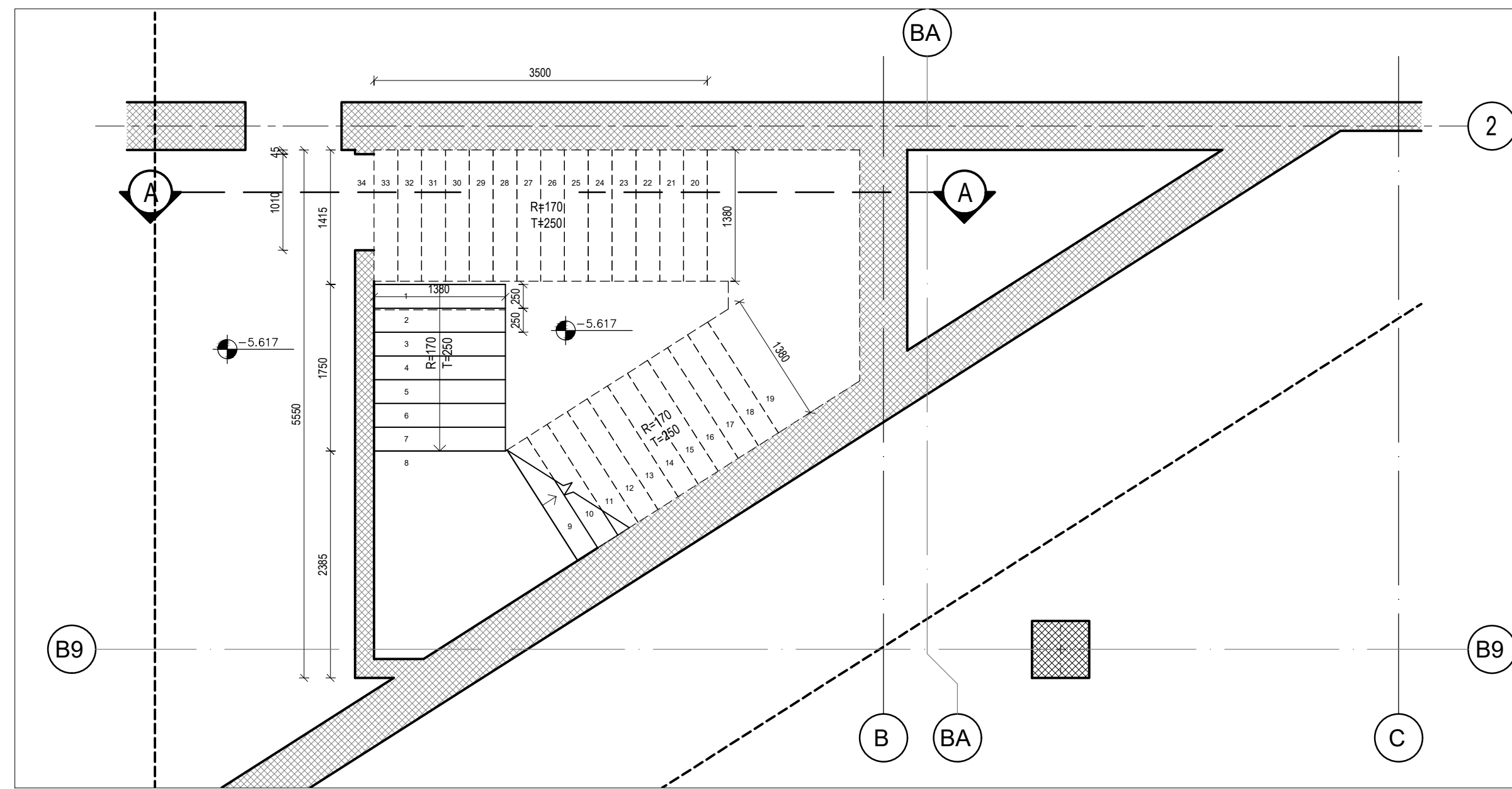
Plani i nivelit f.f. +0.30 Shkalla 1 : 50
